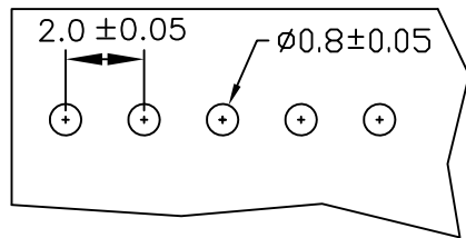
P.C.BOARD LAYOUT
